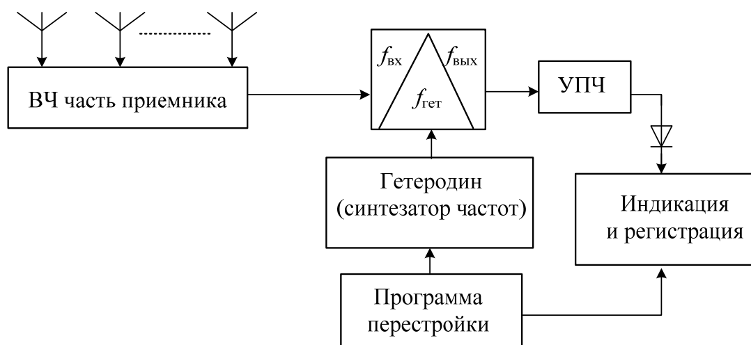
Рис. 1.10.2. Структурная схема современного сканирующего приемника
