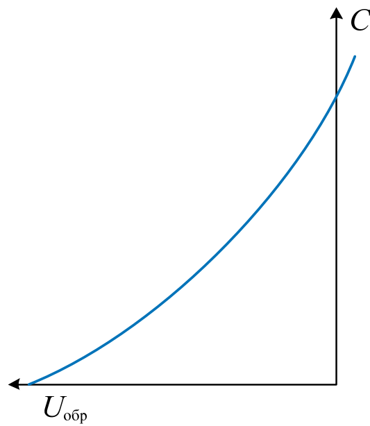
Рис. 2.2.12. Вольт-фарадная характеристика варикапа
