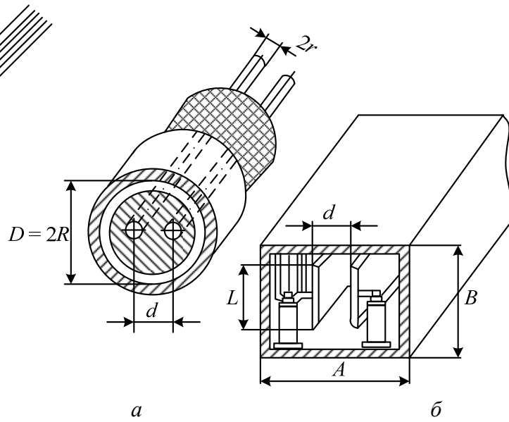
Рис. 3.2.2. Экранированная двухпроводная линия: а – с круглым экраном; б – с ленточными проводниками
