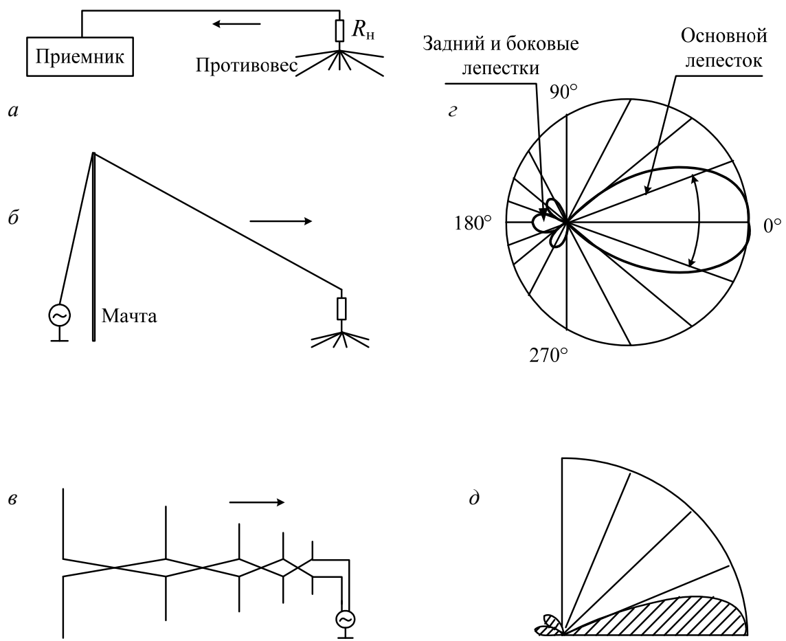
Рис. 3.4.18. Виды антенн и их ДН: a – приемная антенна бегущей волны; б – \lambda -образная передающая антенна бегущей волны; в – логопериодическая антенна; г – ДН в горизонтальной плоскости направленных антенн; д – ДН в вертикальной плоскости направленных антенн
