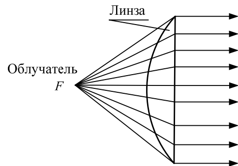
Рис. 3.4.9. Линзовая антенна
