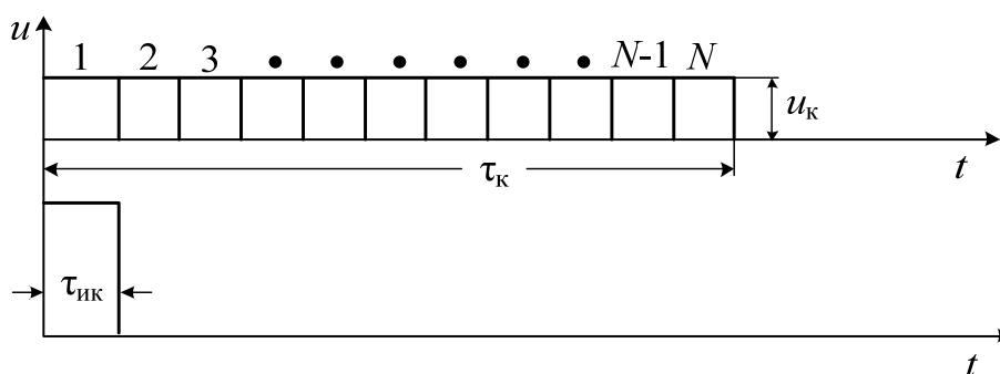
Рис. 1.6.3. Широкополосные сигналы
