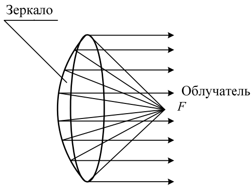
Рис. 3.4.8. Зеркальная антенна
