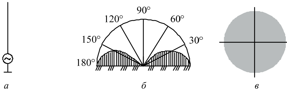
Рис. 3.4.17. Штыревая антенна и ее диаграмма направленности в полярных координатах: a – антенна; б – ДН в вертикальной плоскости; в – ДН в горизонтальной плоскости
