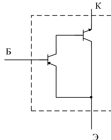
Рис. 2.3.11. Схема Шиклаи
