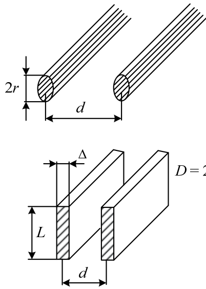
Рис. 3.2.1. Открытая двухпроводная линия
