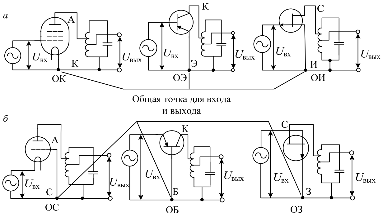
Рис. 3.3.14. Схемы каскадов УРЧ
