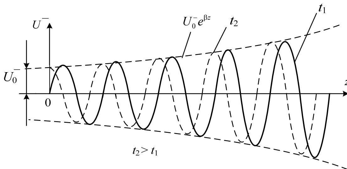
Рис. 3.2.6. Отраженная волна
