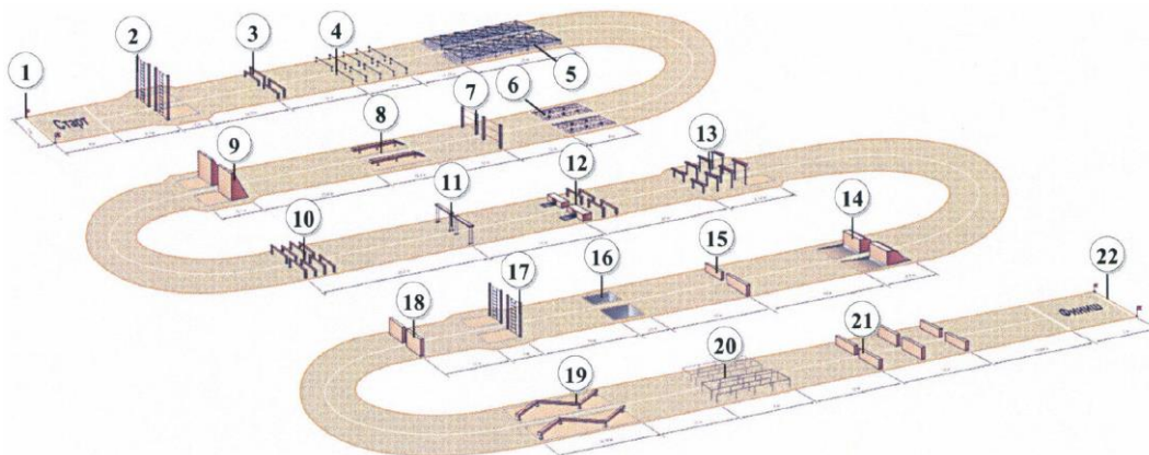
Рис. 49. Схема специальной полосы препятствий
