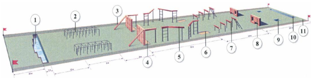
Рис. 43. Схема единой полосы препятствий
