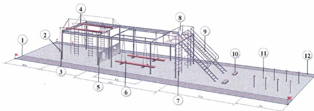
Рис. 47. Схема морской полосы препятствий
