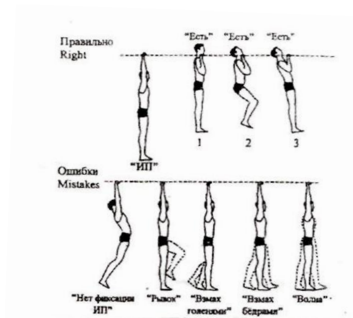
Рисунок 1 – Подтягивание на высокой перекладине
