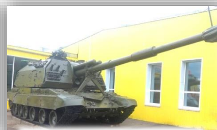
САУ 2С19 «Мста С»
